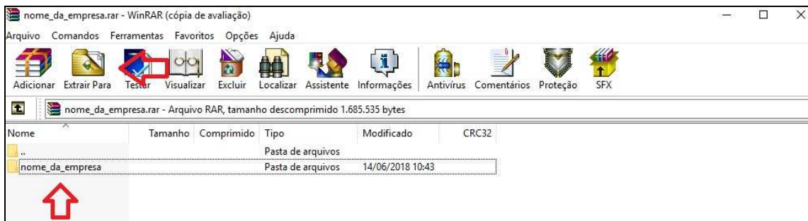
FIGURA 1 – Arquivo .rar
