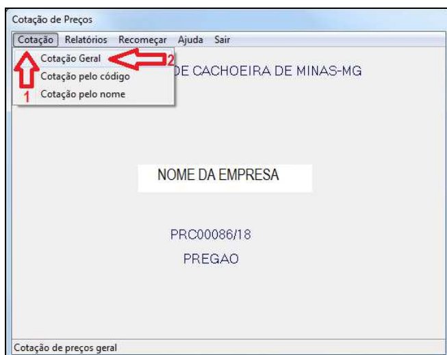
FIGURA 5 – Cotação
