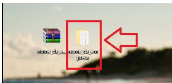
FIGURA 2 – Arquivo extraído
