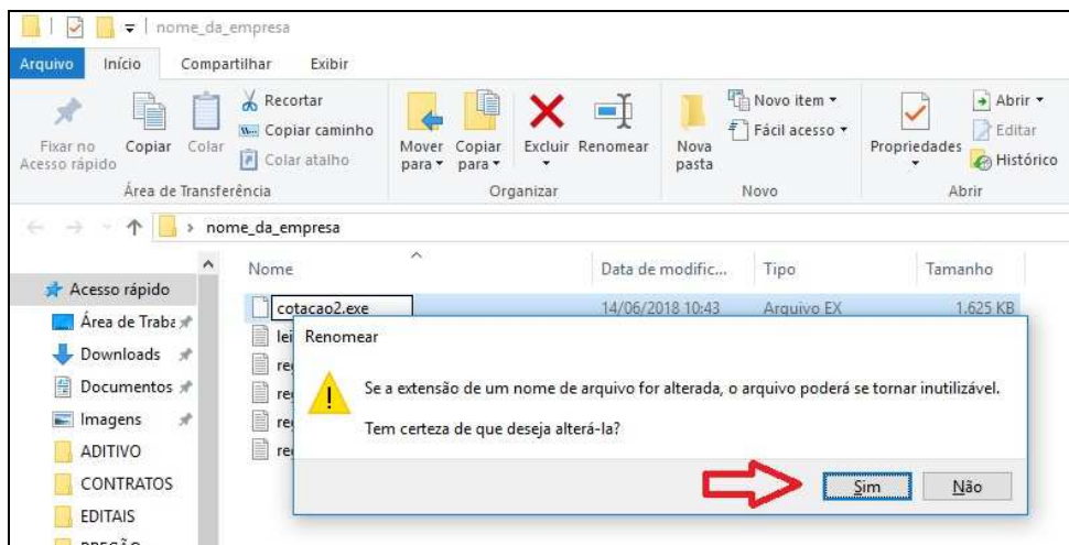
FIGURA 4 – Confirmar alteração
