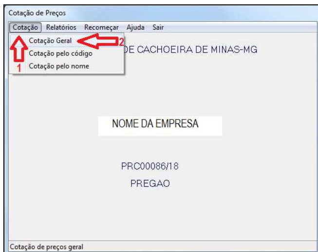
FIGURA 5 – Cotação
